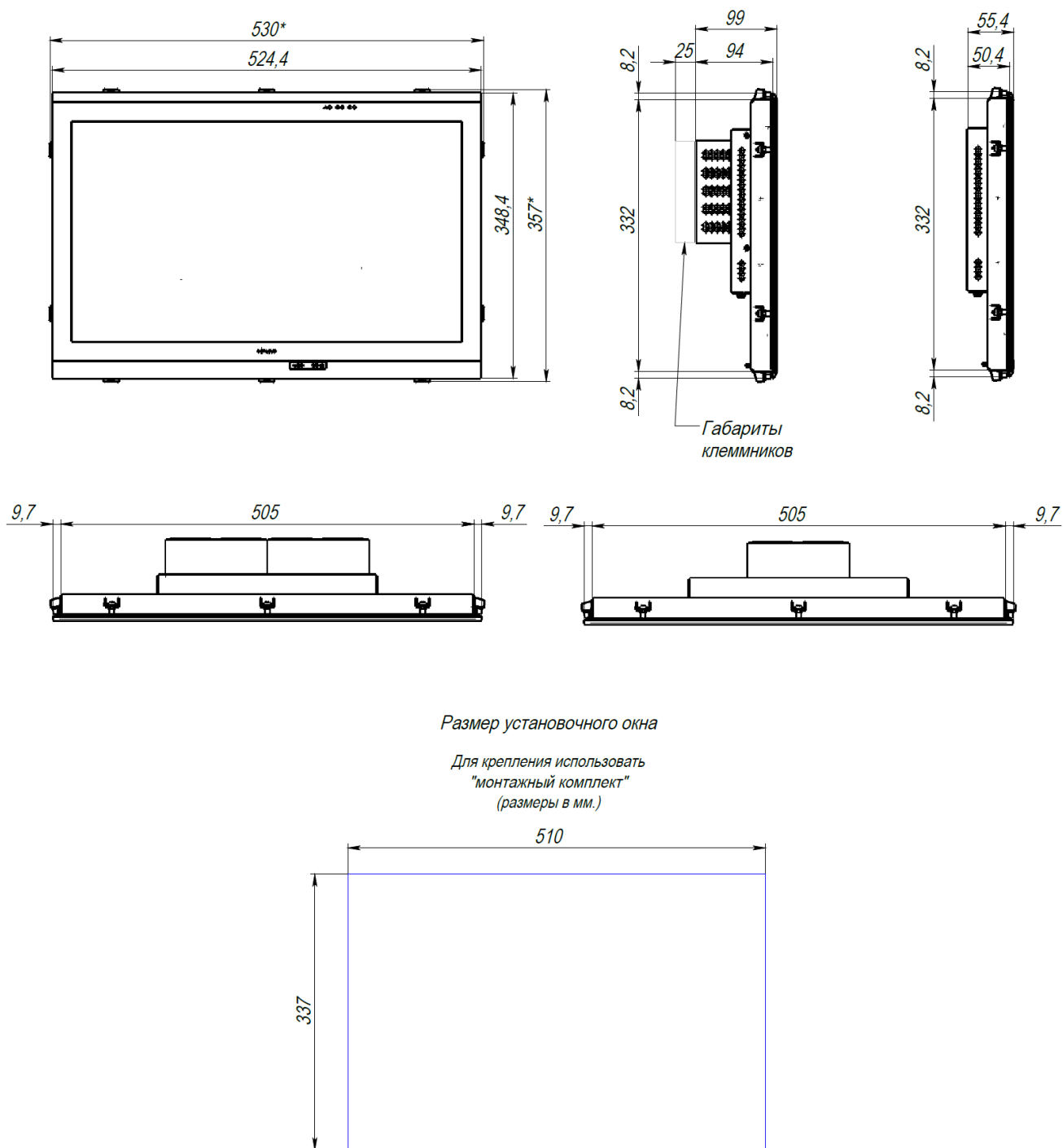
Рисунок П. 9 Габаритные размеры ПО Стабур 21
