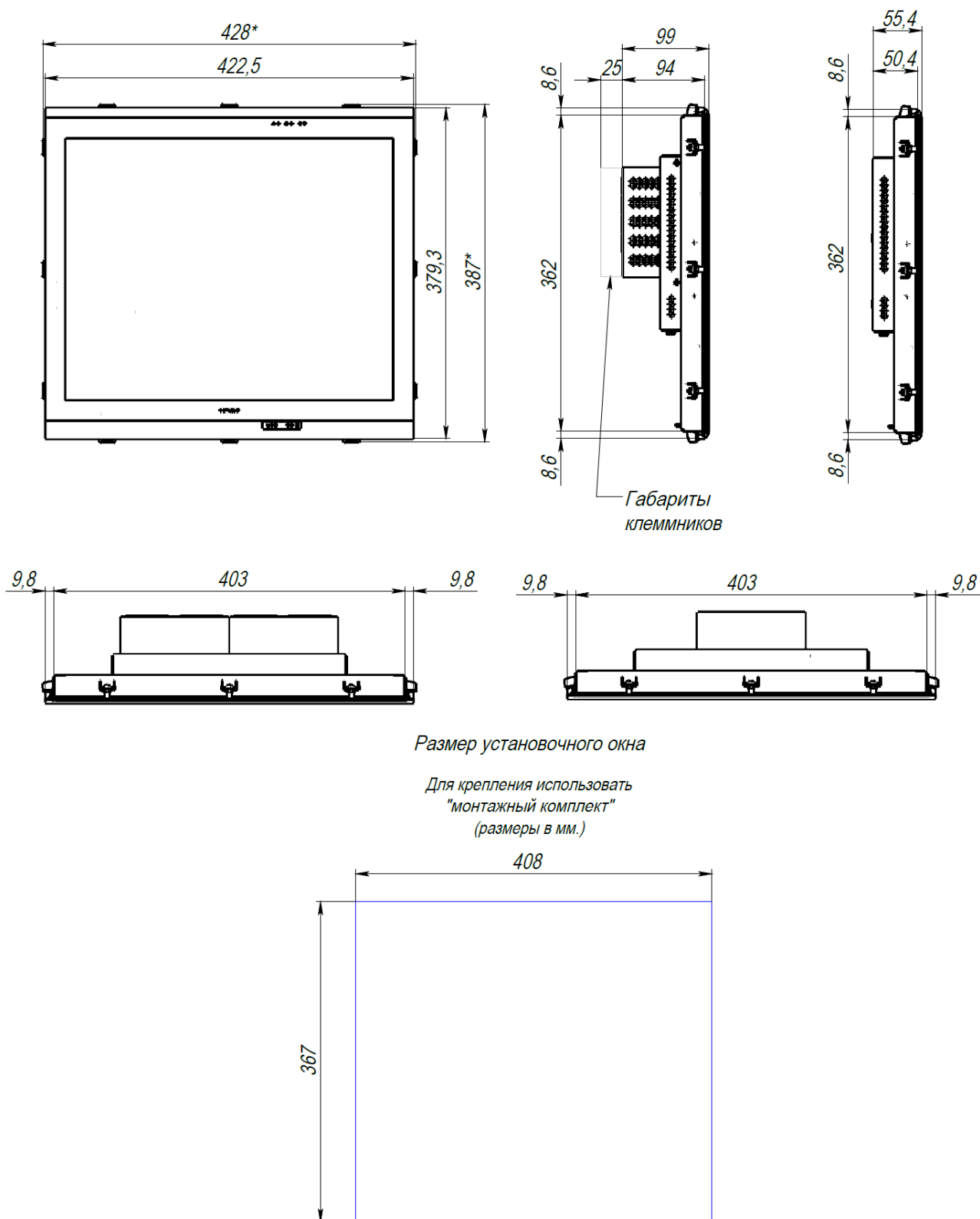
Рисунок П. 8 Габаритные размеры ПО Стабур 19
