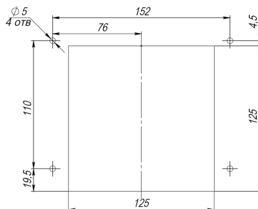
Рисунок П. 2 Габаритные размеры ПО Стабур 07
