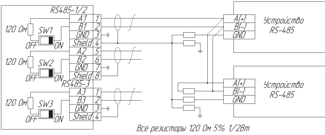
Рисунок П. 12 Схема подключения экранированной линии RS-485 с дренажным проводом к ПО Стабур 10 (в варианте без корзин), 12, 15, 17, 19 и 21
