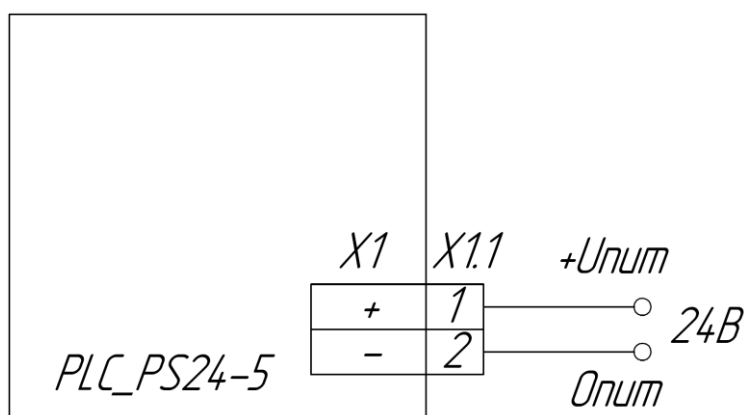
Рисунок 4-7 Схема подключения модуля PS24
