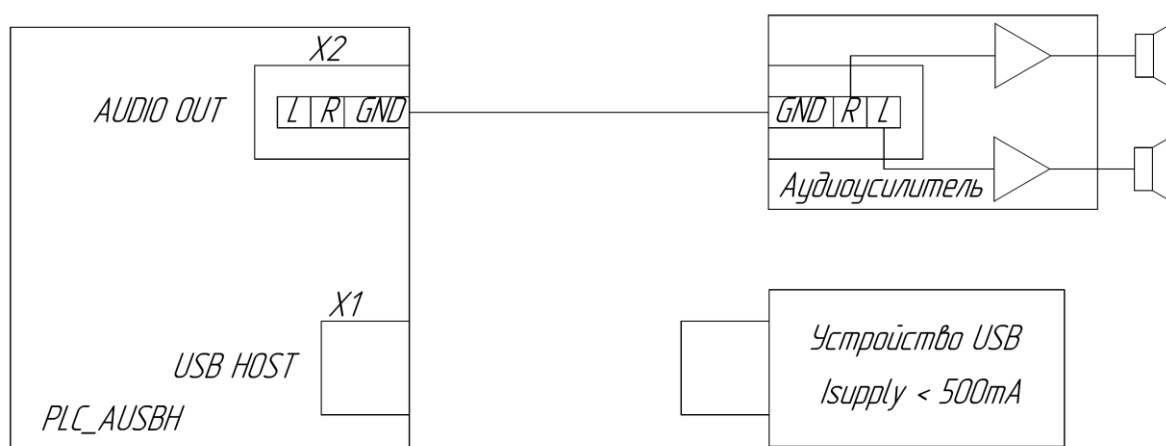
Рисунок 4-6 Схема подключения модуля интерфейсов аудио и USB AUSBH
