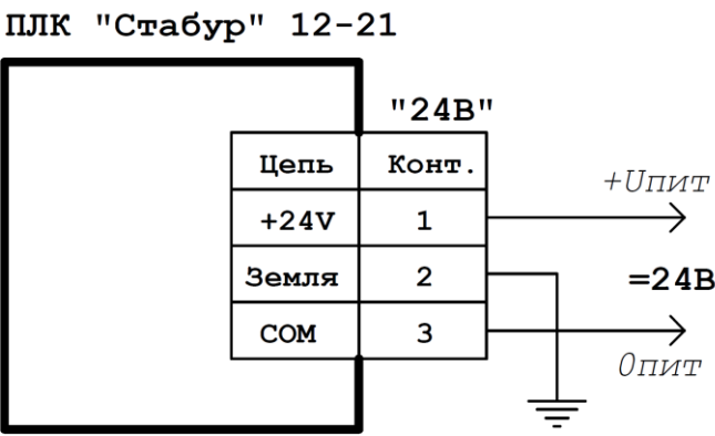
Рисунок П. 10 Схема подключения питания к ПО Стабур 10 (в варианте без корзин), 12, 15, 17, 19 и 21
