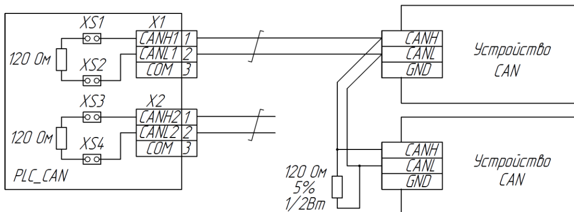
Рисунок 4-4 Схема подключения модуля CAN к линии CAN.
