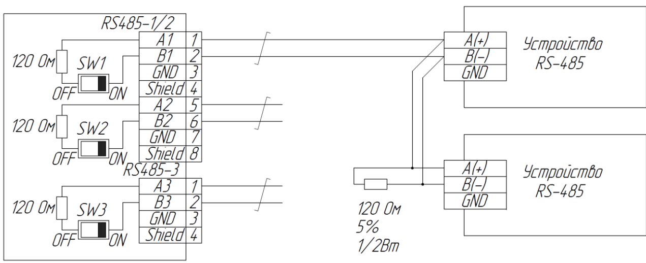
Рисунок П. 11 Схема подключения линии RS-485 к ПО Стабур 10 (в варианте без корзин), 12, 15, 17, 19 и 21
