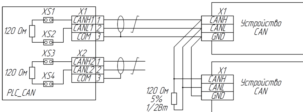
Рисунок 4-5 Схема подключения модуля CAN к экранированной линии CAN с дренажным проводом
