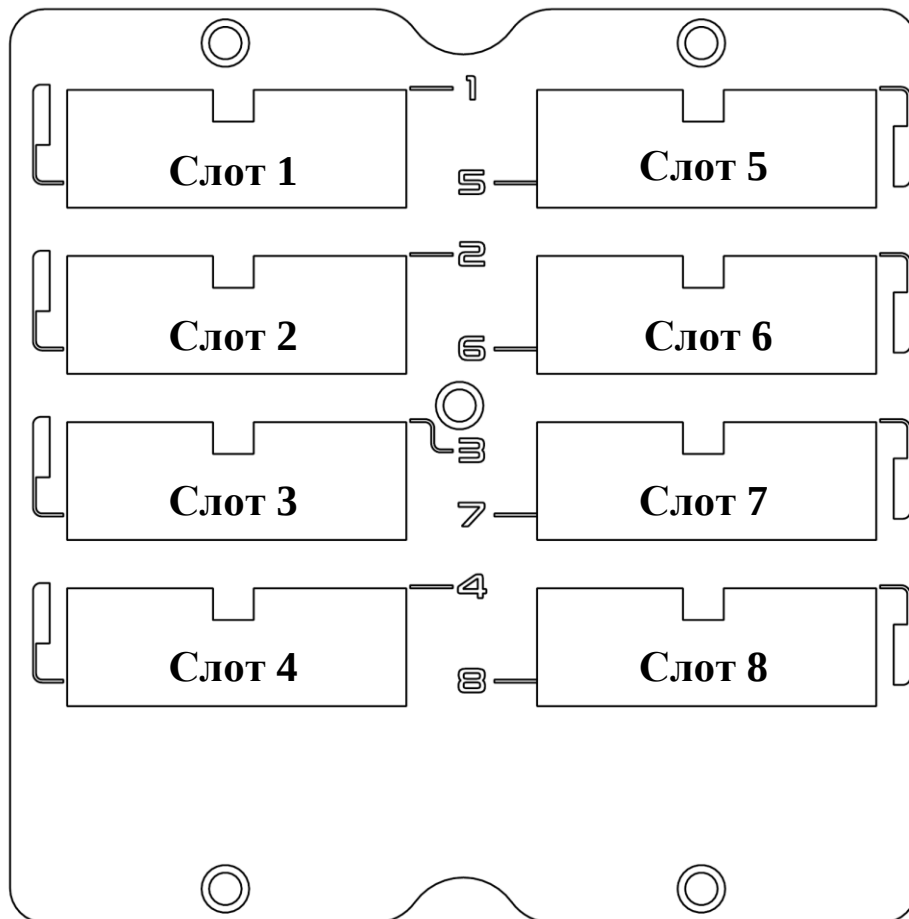
Рисунок 4-1 Нумерация слотов модулей интерфейсов
